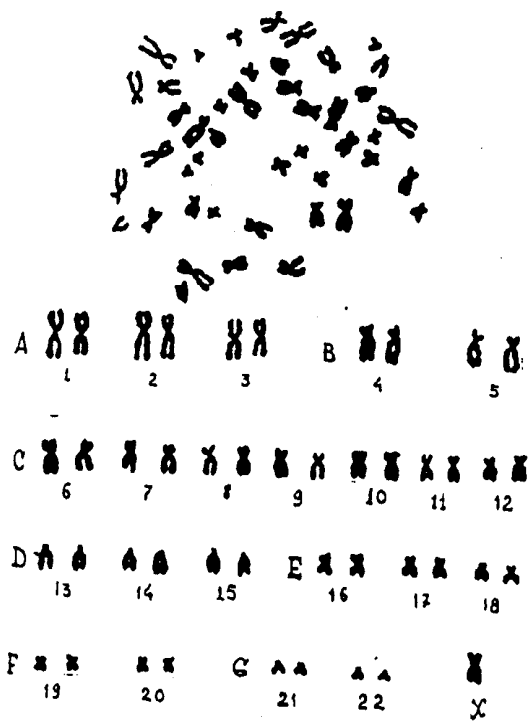
Кариограмма 1.
