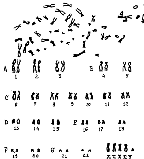
Кариограмма 4.
