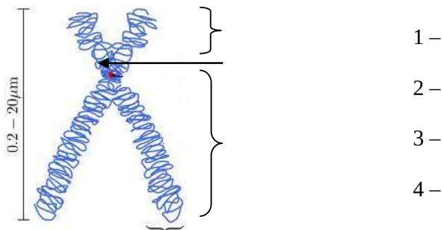
Рис. 1. Метафазная хромосома
