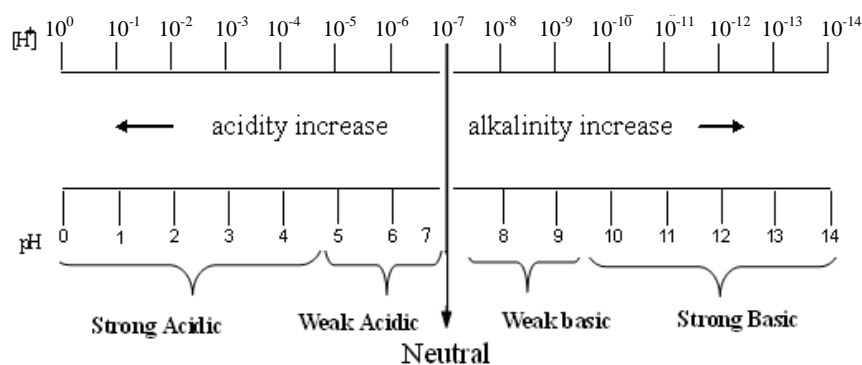
Fig. 6.1. pH scale
